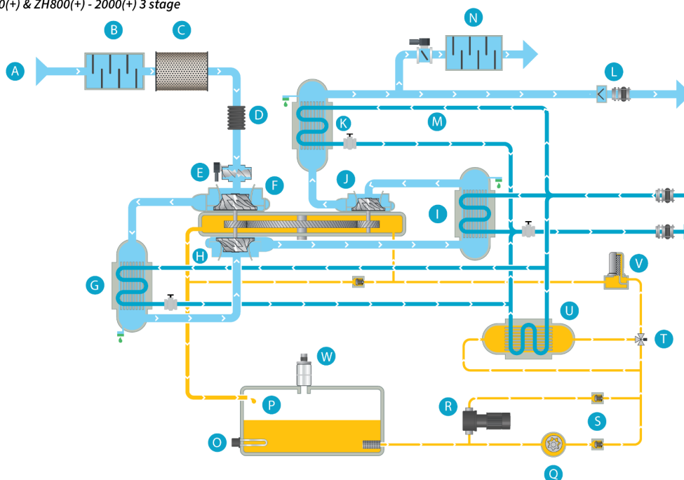
ZH400(+)-1120(+)& ZH800(+)-2000(+) 3 stage
