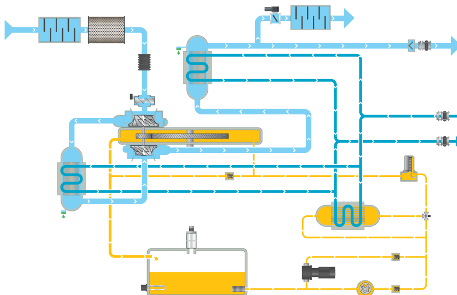
ZH355(+)-800(+)& ZH630(+)-1400(+) 2 stage
